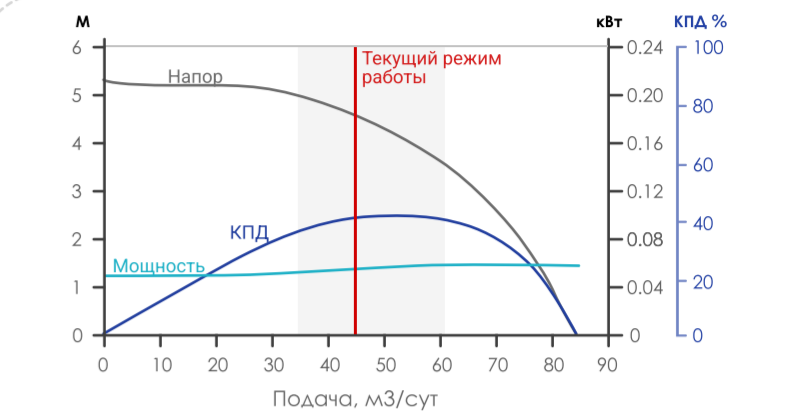
Общая сепарация газа
