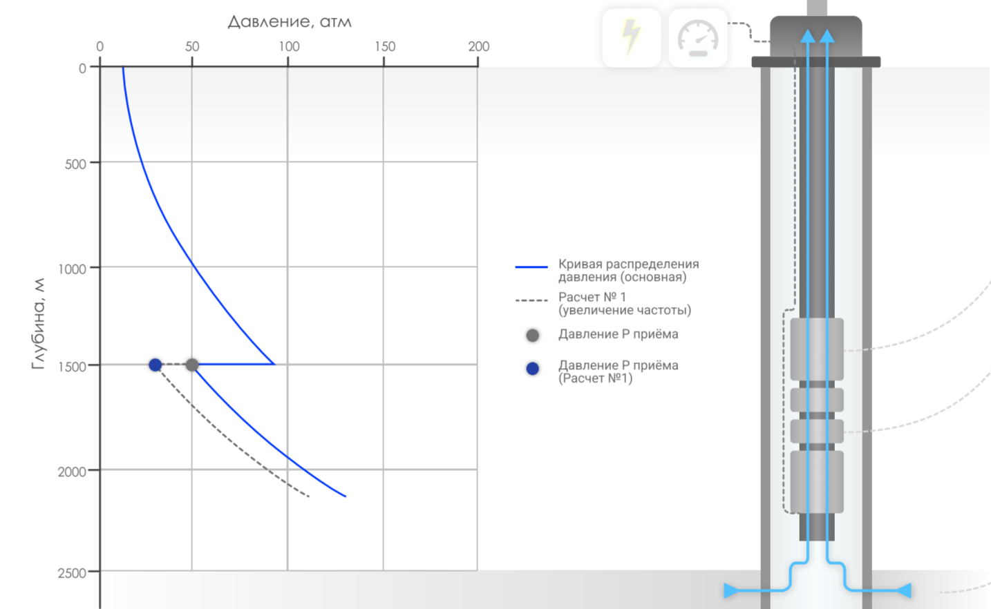
График давления на глубине
