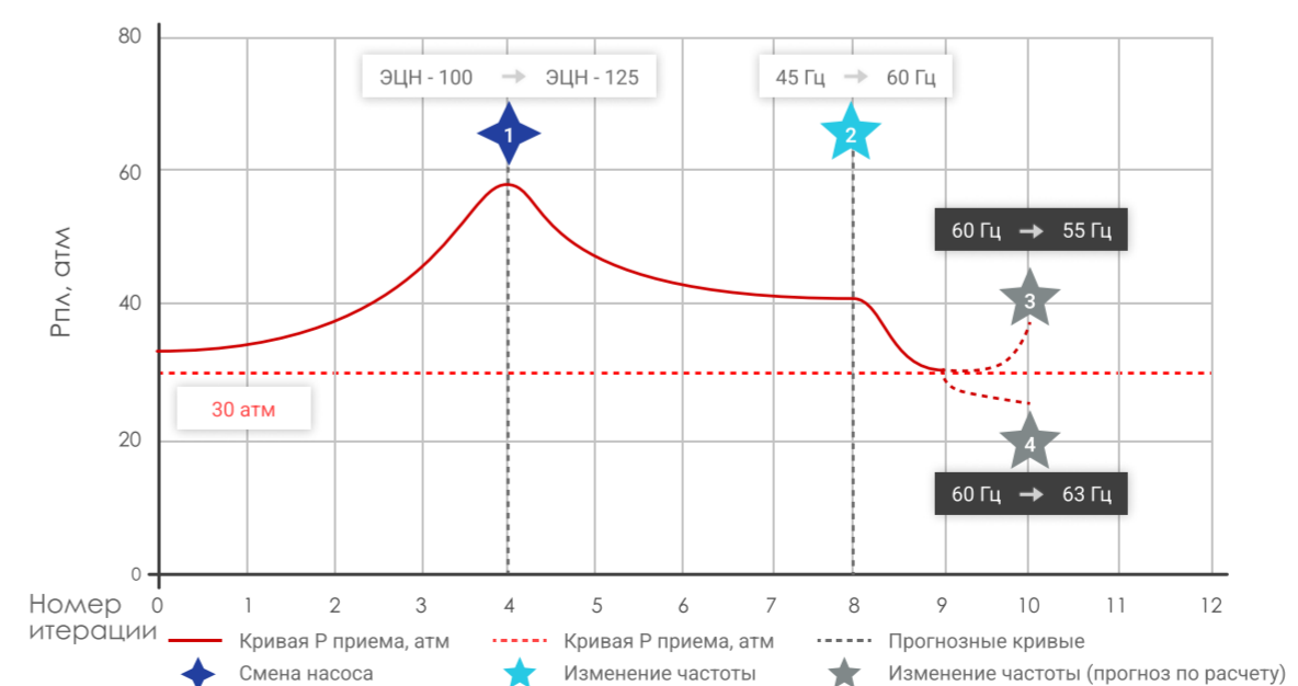
Давление на приеме насоса от времени
